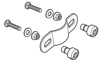
Rod Clamp
